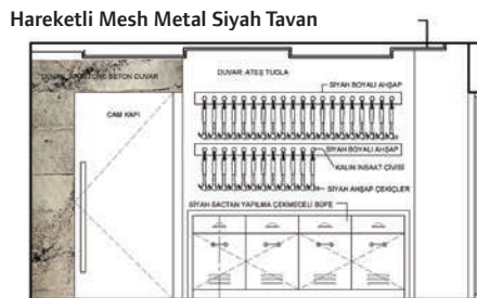
B-B Kesiti
